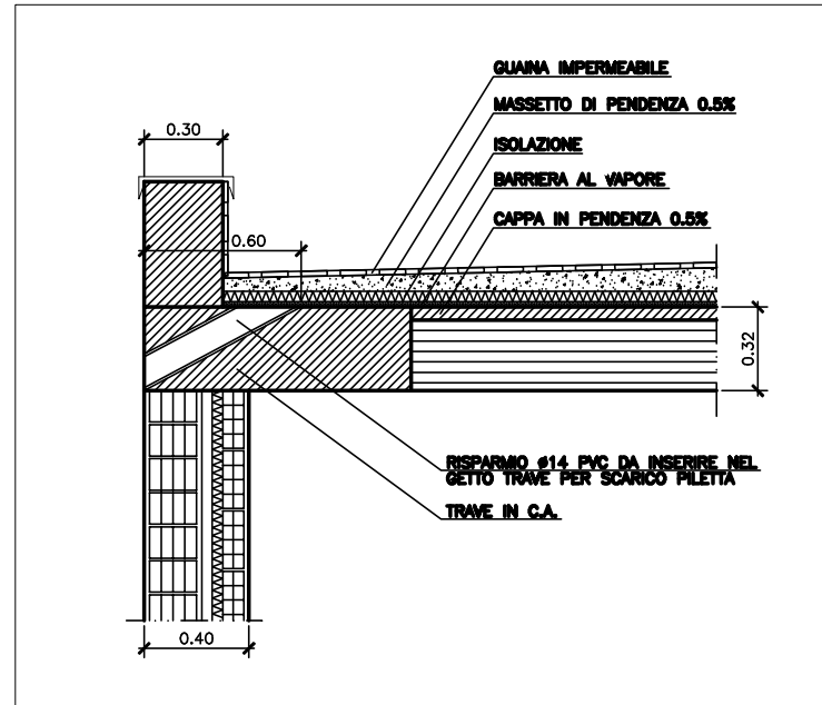
PARTICOLARE COPERTURA IN CORRISPONDENZA DEI CORDOLI PERIMETRALI
