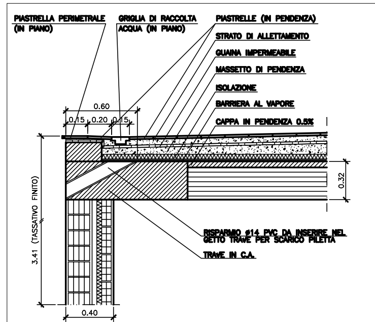
PARTICOLARE COPERTURA IN CORRISPONDENZA DEI TERRAZZI
